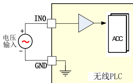
图 3-1 电压档接线图
