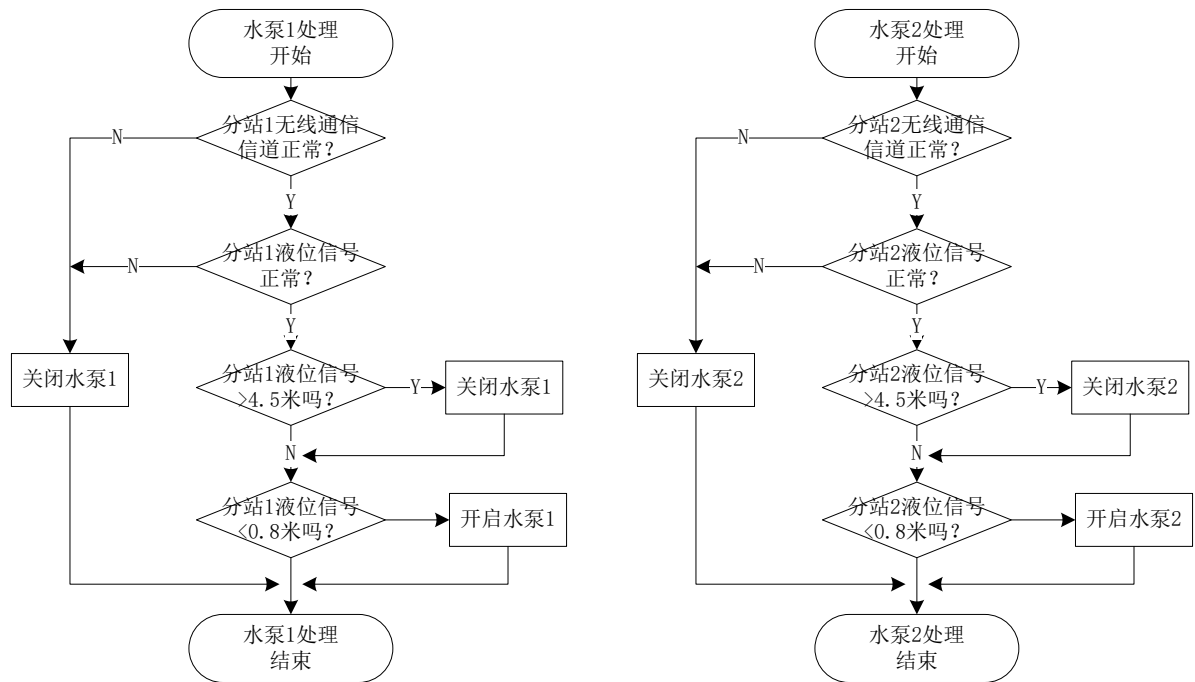
图 7-9 主站程序处理流程图
