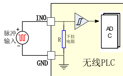
图 3-4 计数档接线图
