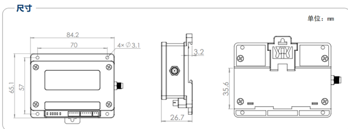
图 2-1T40S 外观尺寸及安装示意图
